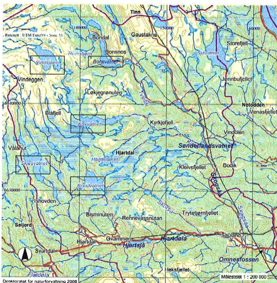
Figur 2.1. Oversiktskart over vassdraget og magasinene i Hjordøla og Skogså (Tuddalsvassdraget).
