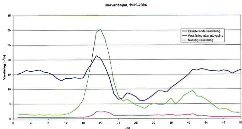
Figur 3. Årsprofil for gjennomsnittlig vannføring nedenfor inntaket til Sauland 1: naturlig vannføring (før utbygging av Hjørdøla kraftverk), eksisterende vannføring (med Hjørdøla kraftverk) og etter utbygging av Sauland kraftverk (Norconsult 2009).
