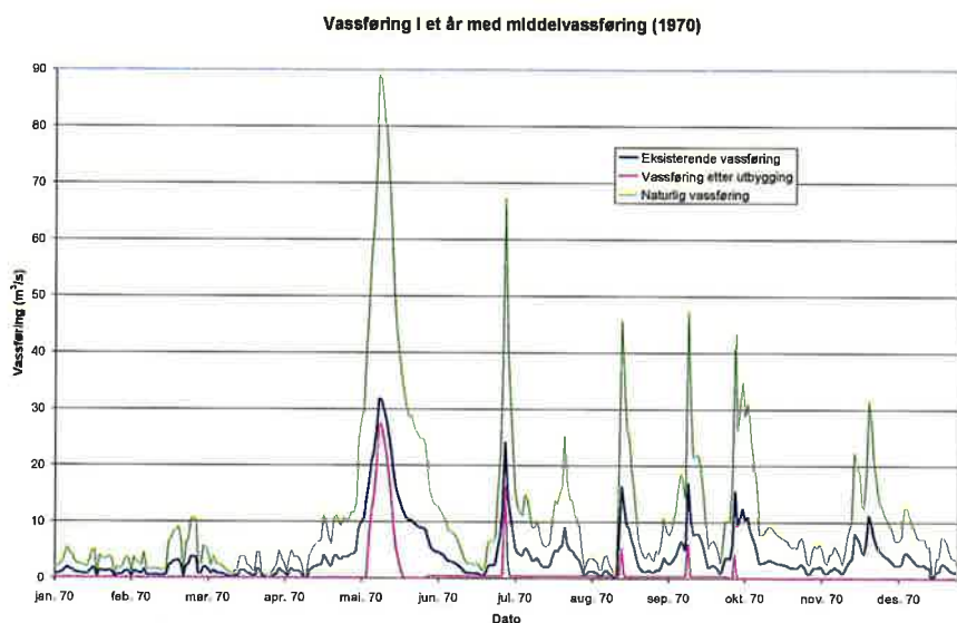
Figur 6. Vannføringsvariasjon nedenfor inntaket til Sauland 2 i året nærmest middelvannføring: naturlig vannføring, eksisterende vannføring (med Hjørdøla kraftverk) og etter utbygging av Sauland kraftverk.
