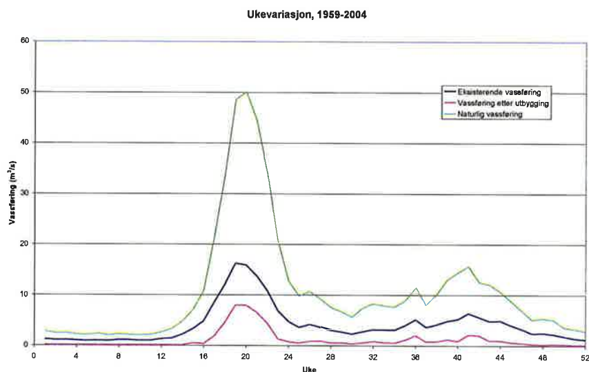
Figur 5. Årsprofiler for gjennomsnittlig vannføring nedenfor inntaket til Sauland 2: naturlig vannføring (før utbygging av Hjørdøla kraftverk), eksisterende vannføring (med Hjørdøla kraftverk) og etter utbygging av Sauland kraftverk (Norconsult, 2009).
