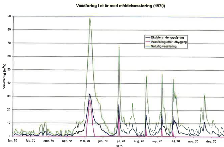
Figur 4 Vannføringsvariasjon nedenfor inntaket til Sauland 2 i året nærmest middelvannføring: naturlig vannføring, eksisterende vannføring (med Hjartdøla kraftverk) og etter utbygging av Sauland kraftverk.
