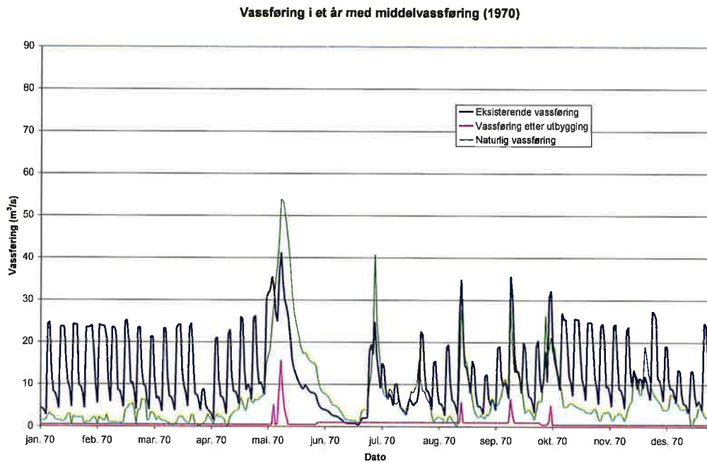
Figur 2 Vannføringsvariasjon nedenfor inntaket til Sauland 1 i året nærmest middelvannføring. Figuren er basert på verdier med døgnoppløsning, slik at de sterke endringene i løpet av uken ved eksisterende vannføring er synlige.
