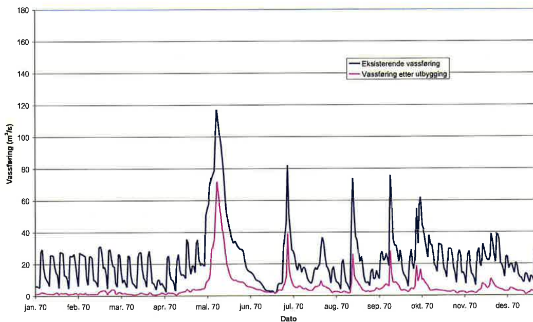
Figur 5 Vannføringsvariasjon ved Omnesfossen umiddelbart oppstrøms utløpet fra Sauland kraftverk i året nærmest middelvannføring, før og etter utbygging.
