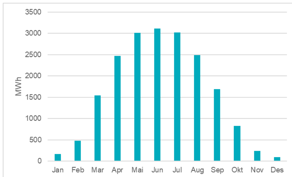
Figur 3-4: Estimert månedlig energiproduksjon
